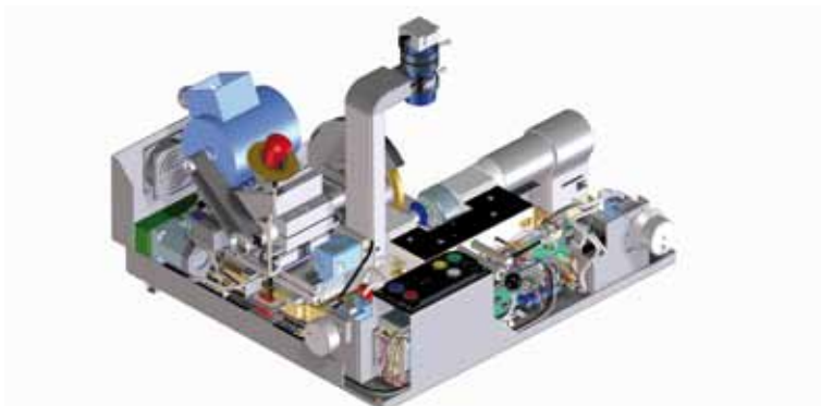
Een diamantslijpmachine.
